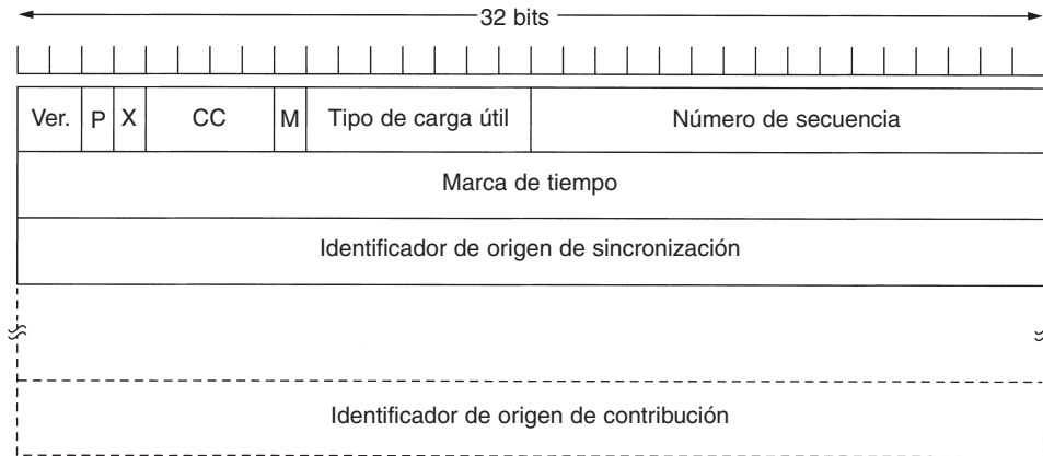
Figura 6-26. El encabezado RTP.
