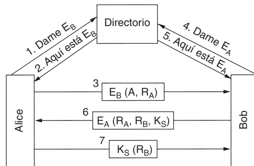
Figura 8-43. Autenticación mutua utilizando la criptografía de clave pública.
