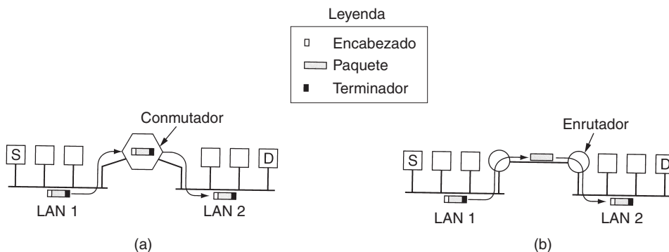
Figura 5-44. (a) Dos Ethernets conectadas mediante un conmutador. (b) Dos Ethernets conectadas mediante enrutadores.
