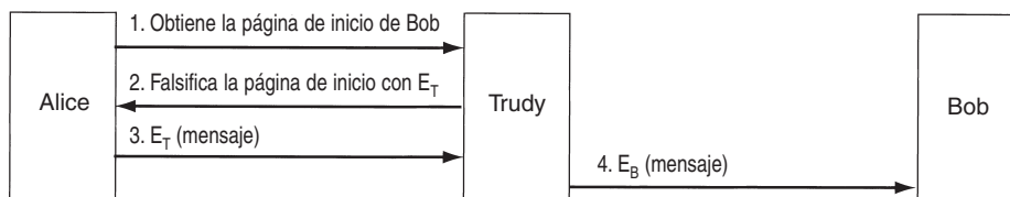
Figura 8-23. Una forma mediante la que Trudy puede subvertir la encriptación de clave pública.
