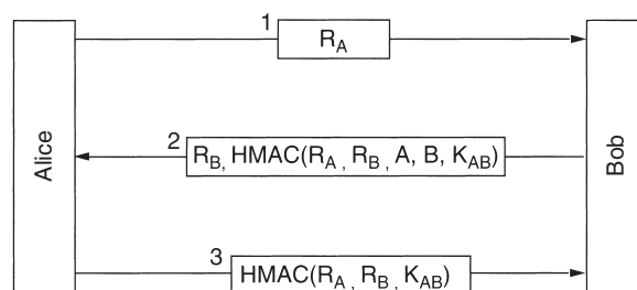
Figura 8-36. Autenticación mediante HMACs.
