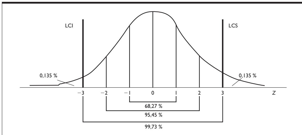
Figura 21.80. Distribución normal.
