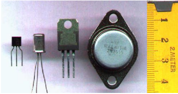
Figura 1.3: Transistores
