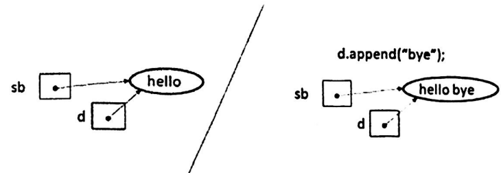
Fig. 6-4. Paso de parámetros de tipo objeto
