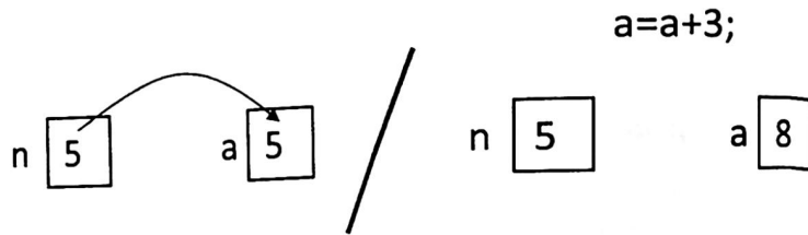
Fig. 6-3. Paso de parámetros de tipos primitivos
