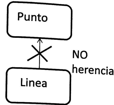
Fig. 7-4. Caso incorrecto de herencia
