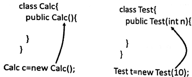
Fig. 6-6. Ejecución de constructor
