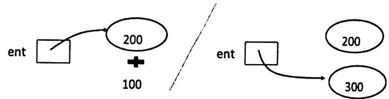
Fig. 2-10. Inmutabilidad de objetos de envoltorio
