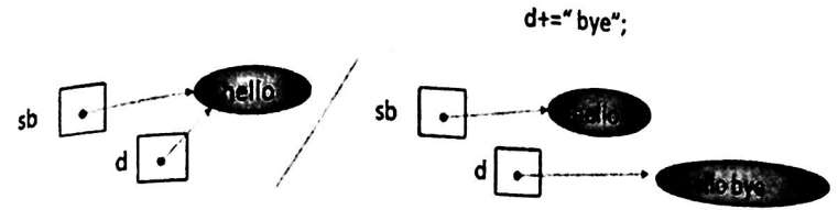
Fig. 6-5. Parámetros tipo String
