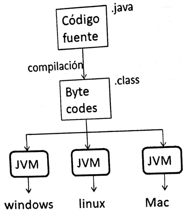
Fig. 1-2. La Máquina Virtual Java
