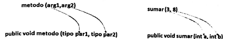
Fig. 6-1. Paso de parámetros a métodos
