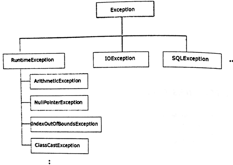
Fig. 8-1. Clases de excepciones
