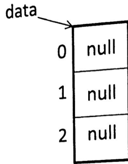
Fig. 4-4. Inicialización por defecto de la primera dimensión
