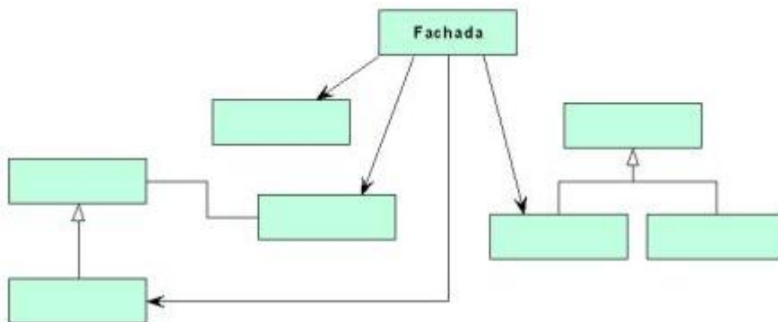
Ilustración 115: Facade
