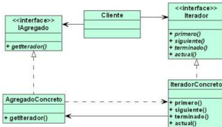
Ilustración 121: Iterator
