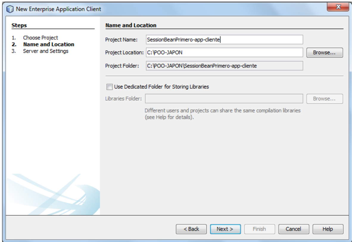
Ilustración 82: Nombre aplicación
