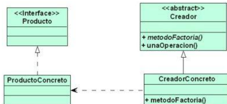
Ilustración 107: Factory Method
