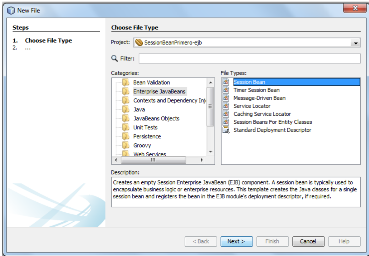
Ilustración 89: Seleccionar SessionBean
