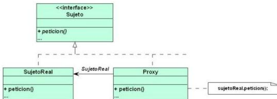
Ilustración 117: Proxy
