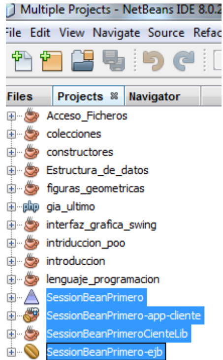
Ilustración 86: Proyecto creados
