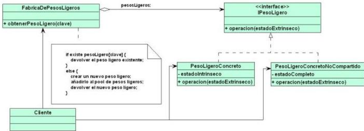
Ilustración 116: Flyweight
