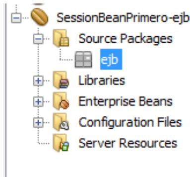
Ilustración 87: Crear Paquete
