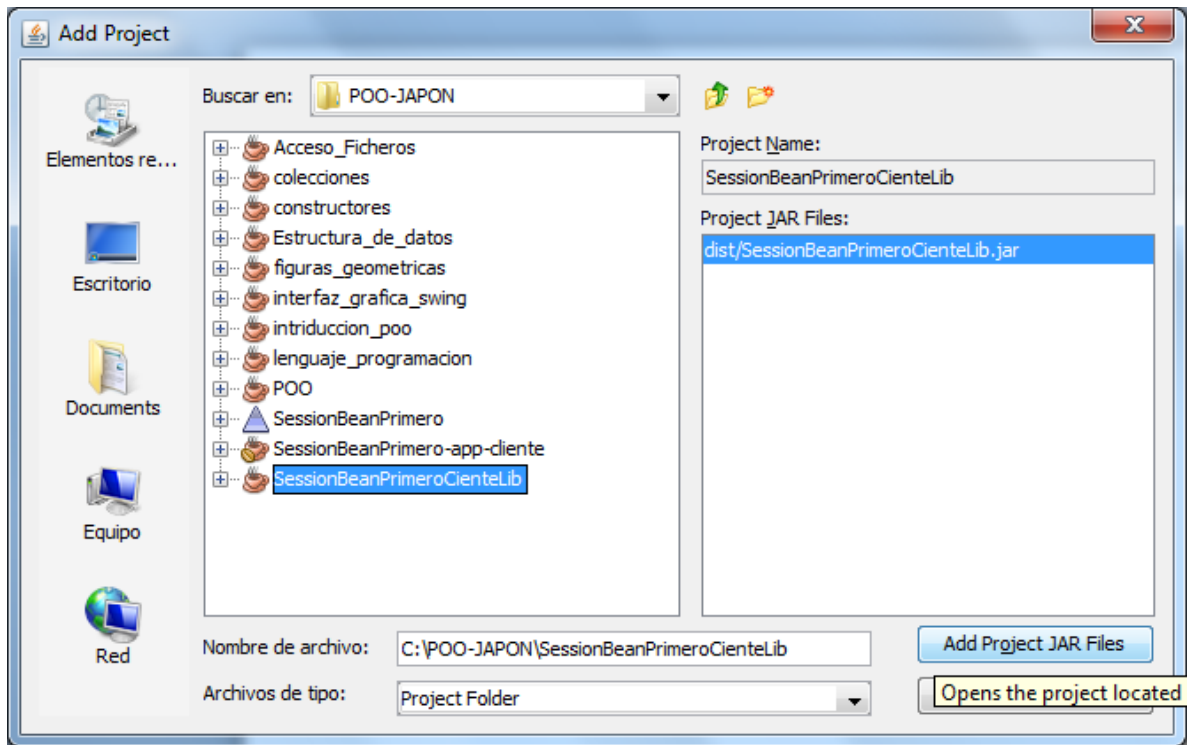
Ilustración 98: Buscar proyecto
