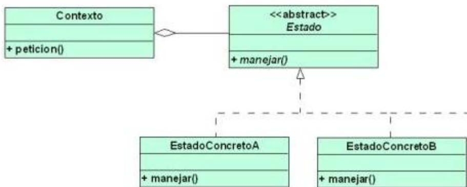
Ilustración 124: State
