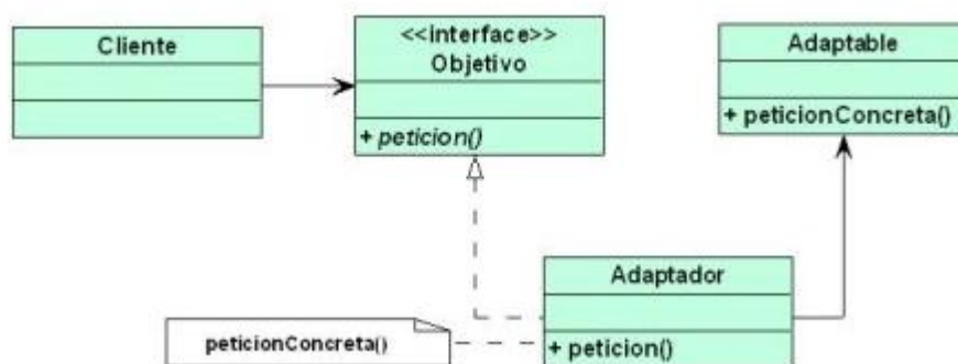
Ilustración 111: Adapter
