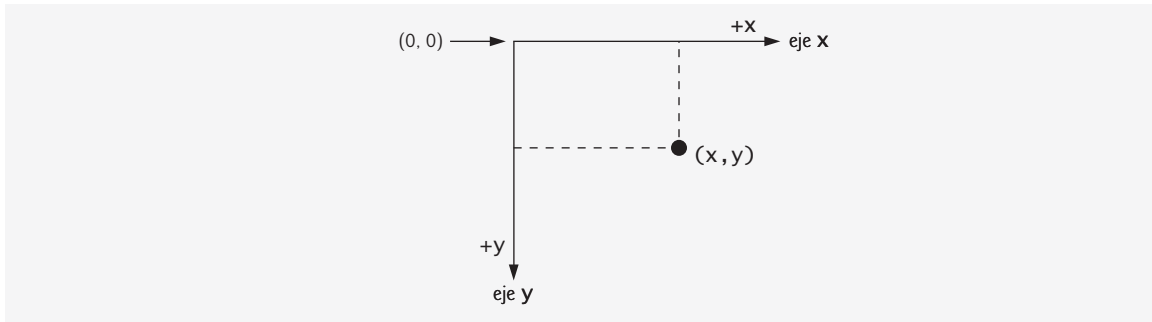
Figura 12.2 | Sistema de coordenadas de Java. Las unidades se miden en píxeles.
