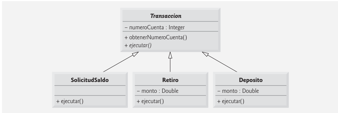
Figura 10.20 | Diagrama de clases que modela la generalización de la superclase Transaccion y las subclases SolicitudoSaldo , Retiro y Deposito . Observe que los nombres de las clases abstractas (por ejemplo, Transaccion ) y los nombres de los métodos (por ejemplo, ejecutar en la clase Transaccion ) aparece en cursivas.
