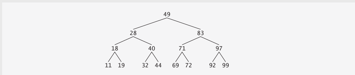
Figura 17.20 | Árbol de búsqueda binaria con 15 nodos.
