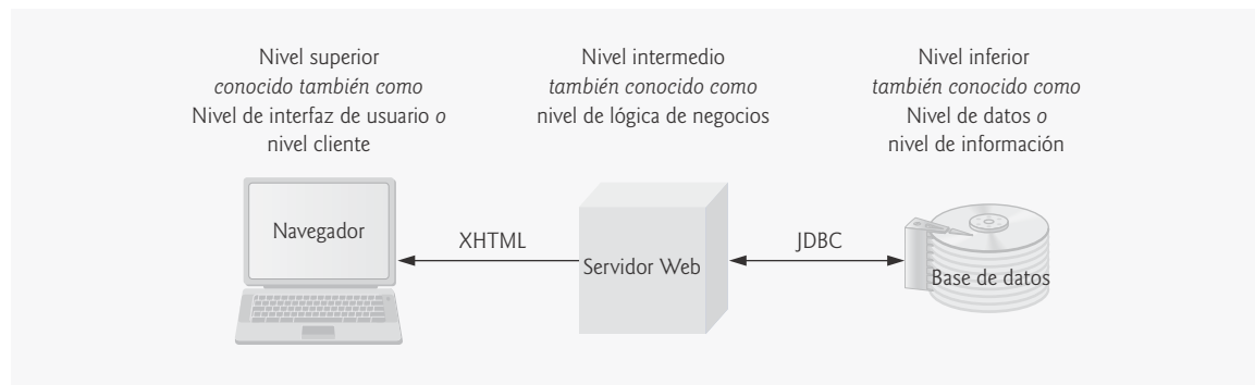
Figura 26.3 | Arquitectura de tres niveles.
