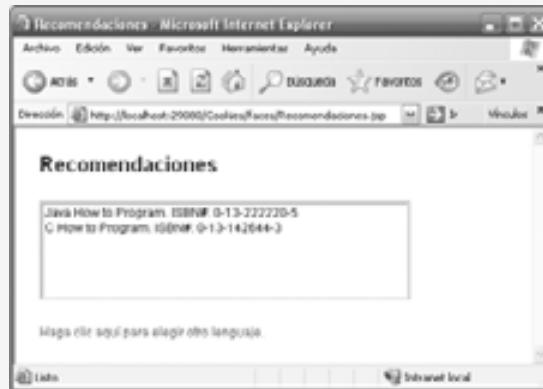
Figura 26.23 | Archivo de JSP que muestra las recomendaciones de libros, con base en cookies. (Parte 2 de 2).
