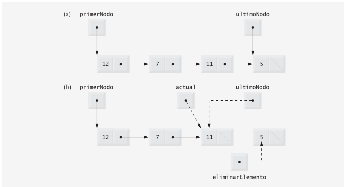
Figura 17.9 | Representación gráfica de la operación eliminarDeFinal .
