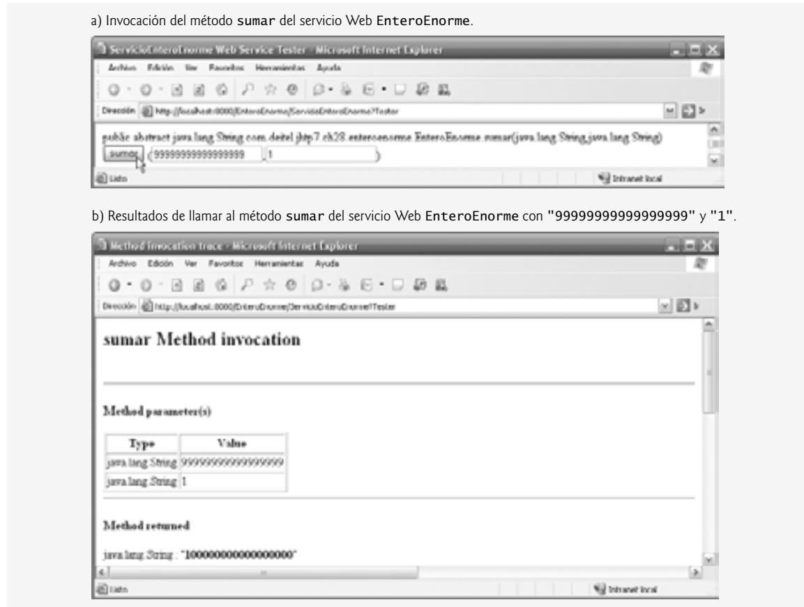
Figura 28.5 | Prueba del método sumar de EnteroEnorme .
