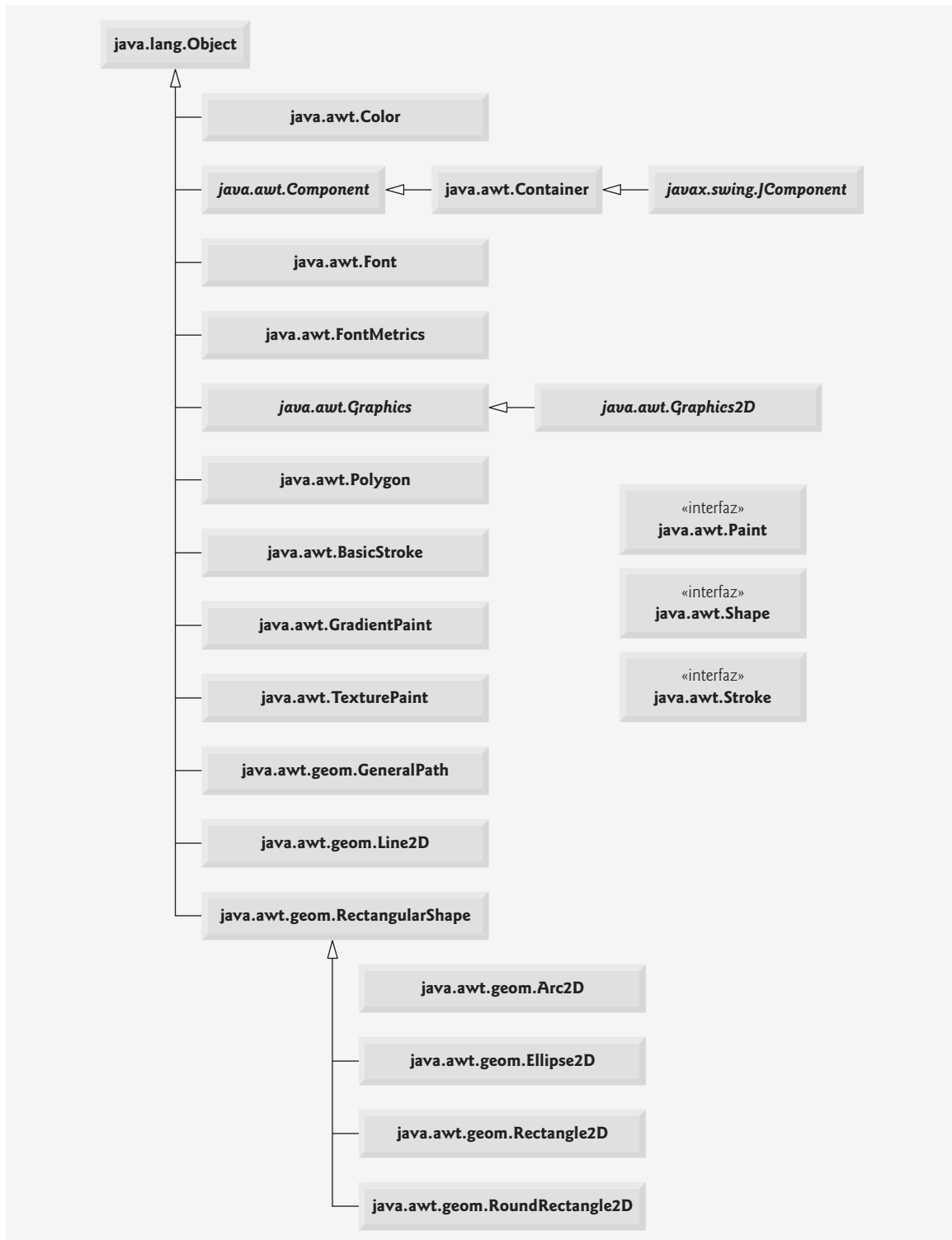
Figura 12.1 | Clases e interfaces utilizadas en este capítulo, provenientes de las herramientas de gráficos originales de Java y de la API Java2D. [Nota: la clase Object aparece aquí debido a que es la superclase de la jerarquía de clases de Java. Además, las clases abstract aparecen en cursiva].
