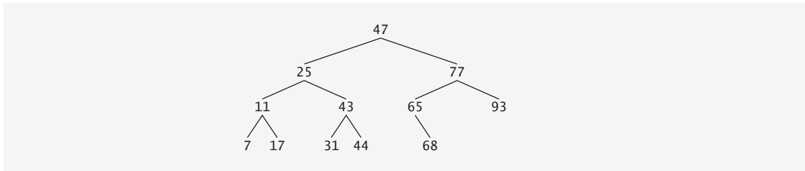
Figura 17.16 | Árbol de búsqueda binario que contiene 12 valores.
