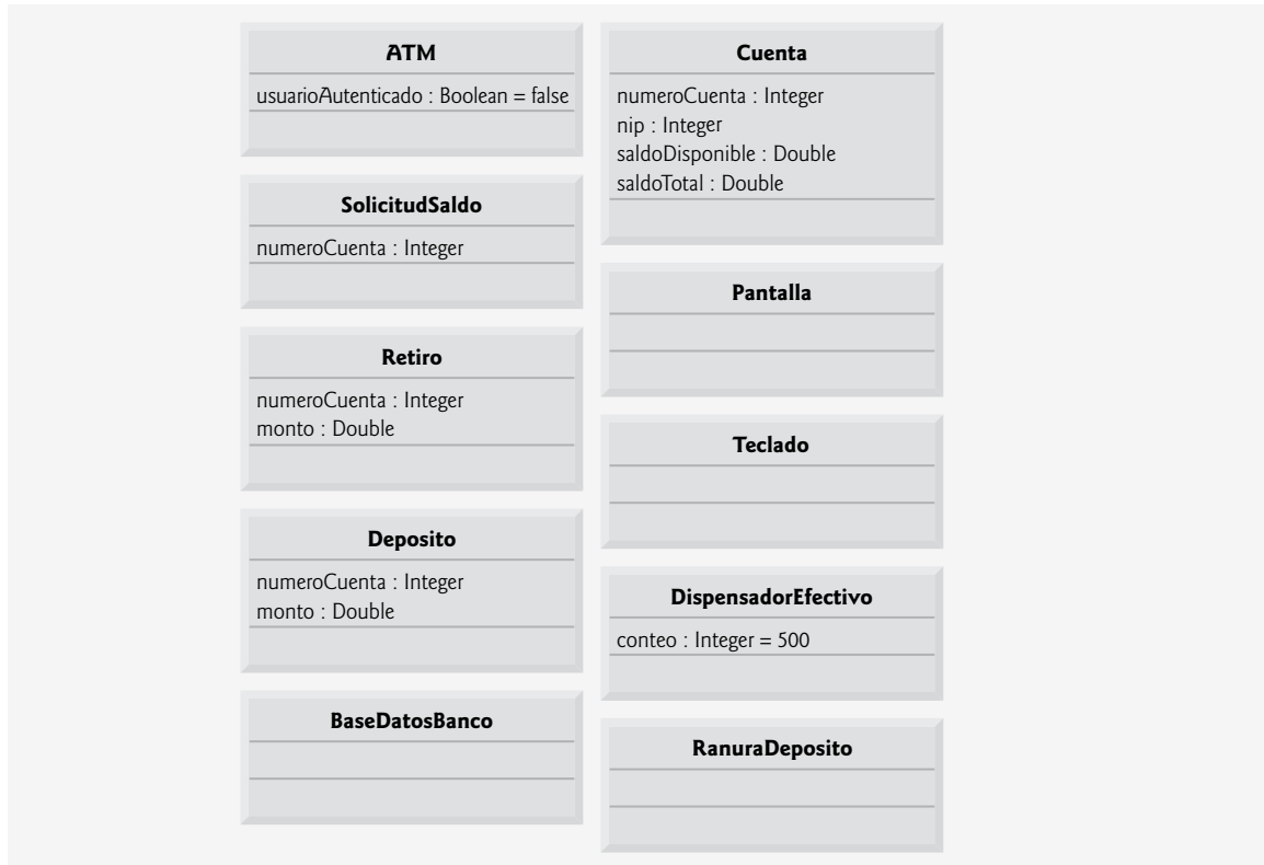
Figura 4.24 | Clases con atributos.
