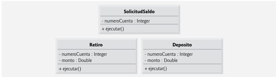
Figura 10.19 | Atributos y operaciones de las clases SolicitudSaldo , Retiro y Deposito .
