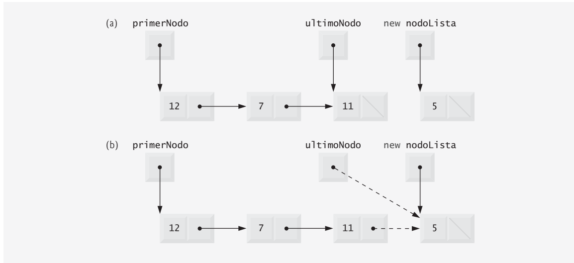
Figura 17.7 | Representación gráfica de la operación insertarAlFinal .
