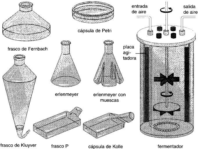
Fig. 6.5 Recipientes para el cultivo superficial y sumergido de microorganismos aerobios.
