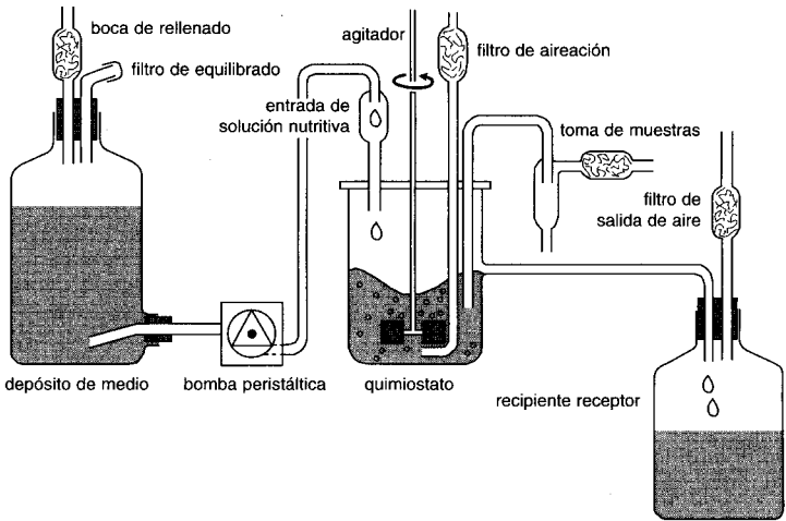
Fig. 6.12 Principio del cultivo continuo en un quimiostato.
