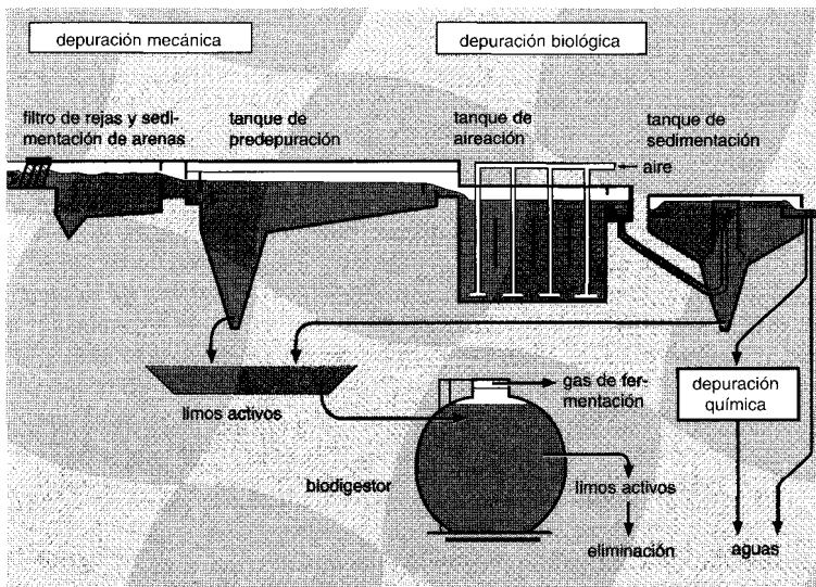
Fig. 17.4 Esquema de una depuradora para limpiar mecánica y biológicamente aguas residuales.
