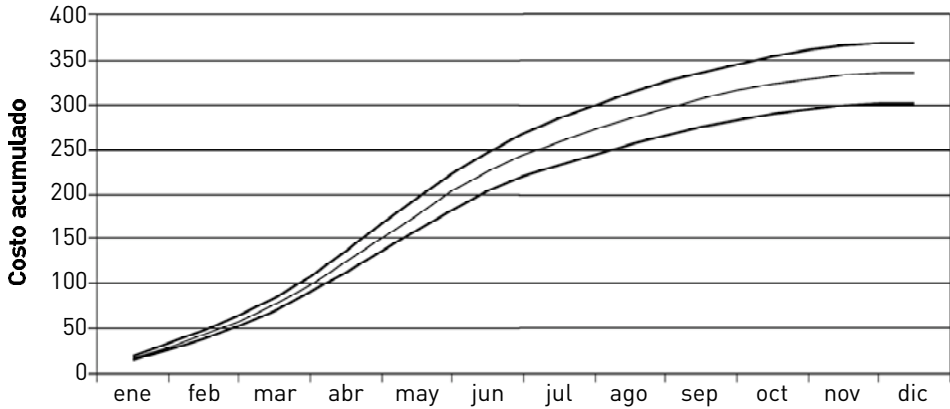
Gráfico 10.3 Autopista base
