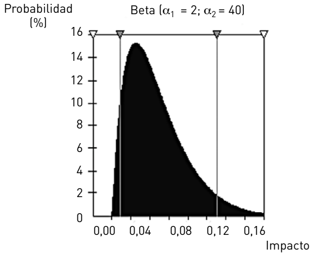
Gráfico 21.7 Distribución beta
