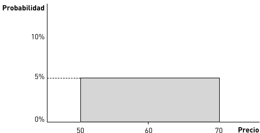
Gráfico 21.4 Distribución uniforme
