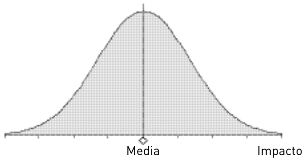
Gráfico 21.8 Distribución normal
