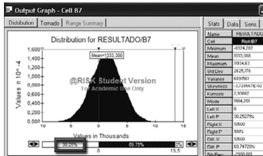
Gráfico 32 Risk 13
